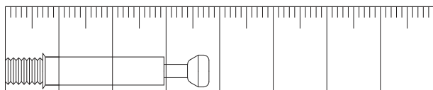
① : Cam Bolt (φ6*35mm) x 20
