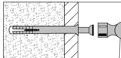
Kołek ścienny nr 5 „Mocowanie młotkiem”.
