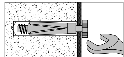
Nr.6 "Shield Anchor" muurplug Zware belasting
