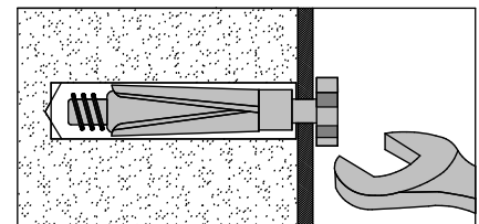
Cheville murale n°6 « Shield Anchor» Charge lourde
