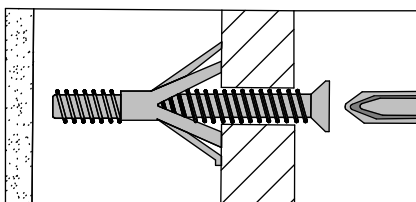
Kołek ścienny nr 3 „Mocowanie wewnętrzne”.
