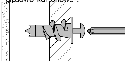
Kołek ścienny nr 2 „Płyta gipsowo-kartonowa”.
