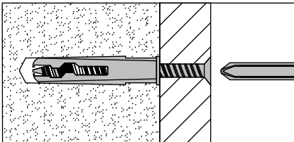
Nr.1 "General Purpose"-wandstekker
