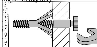
Kołek ścienny nr 4 „Mocowanie wewnętrzne – Heavy Duty”.
