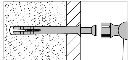
Taco de pared n.º 5 "Fijación de martillo"
